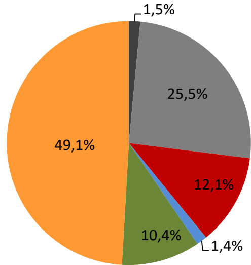
Energieträgermix Deutschland
